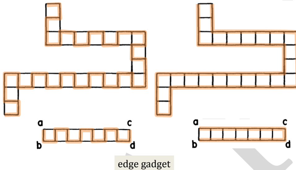
Figure 4.5: Edge gadget.
